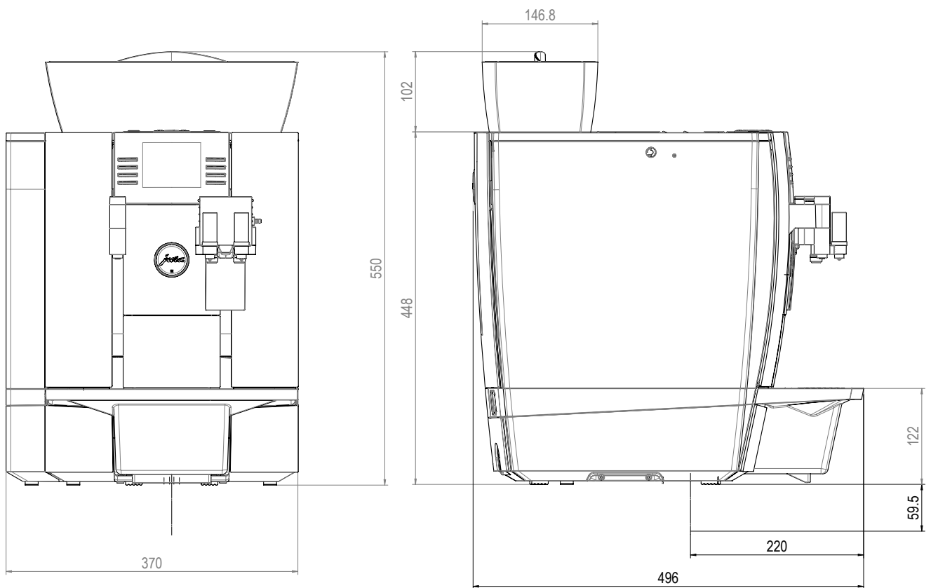
Aufriss
